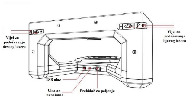
Slika 7. MakerBot Digitizer stražnja strana [5]
