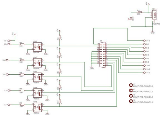
Slika 3. Elektronička shema sklopa za komunikaciju s paralelnim portom računala
