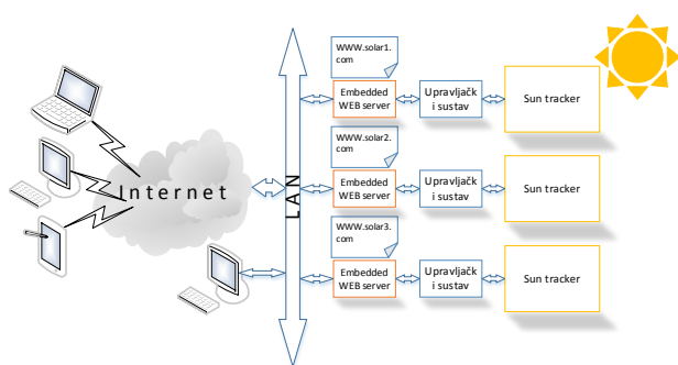
Slika 5. Blok shema sustava s ugradbenim WEB serverom.
