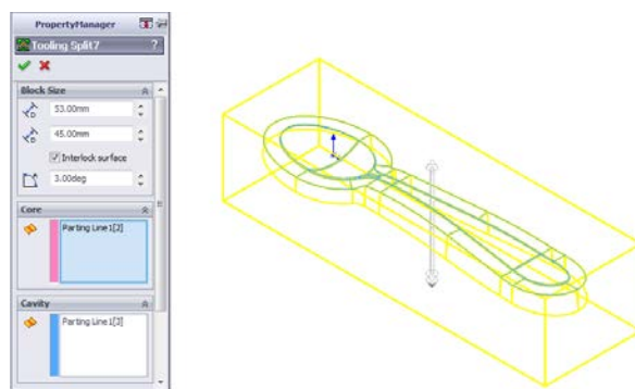
Slika 9. Opcija Tooling Split
