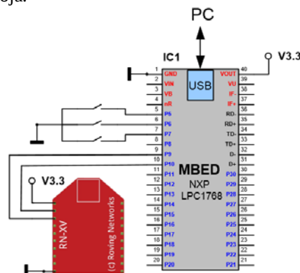
Slika 12. Shema spoja MBED-a i Wi-Fly modula.
